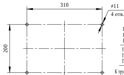
Разметка для крепления газоанализатора
