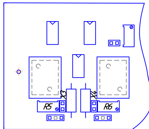
б) плата аналоговая ДАТ-М-02/-04;
