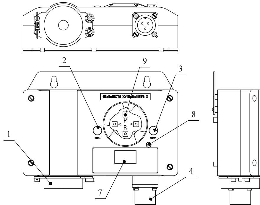
а) сигнализаторы ДАТ-М-01;
