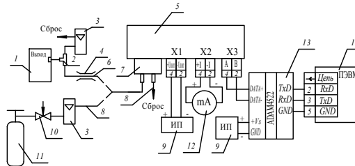
ж) для газоанализаторов ДАХ-M-06TR-H 2 S-40, ДАХ-M-06TR-RSH-5, ДАХ-M-06TR-SO 2 -20, ДАХ-M-06TR-Cl 2 -25, ДАХ-M-06TR-Cl 2 -50, ДАХ-M-06TR-NO 2 -10, ДАХ-M-06TR-N 2 O 4 -20, ДАХ-M-06TR-HCl-30
