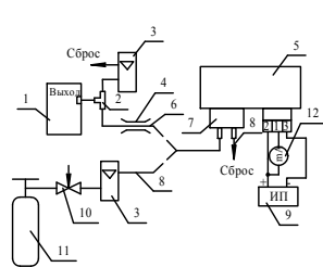
б) для газоанализаторов ДАХ-M-04-H 2 S-40, ДАХ-M-04-SO 2 -20, ДАХ-M-04-Cl 2 -25, ДАХ-M-04-Cl 2 -50, ДАХ-M-04-NO 2 -10, ДАХ-M-04-N 2 O 4 -20, ДАХ-M-04-HCl-30, ДАХ-M-04-RSH-5
