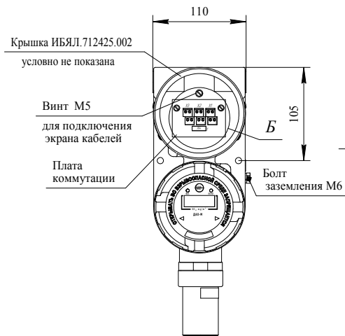
в) газоанализаторы ДАХ-М-05/-05X/-05XH/-06/-06TP/-06TPX/-06TPXH
