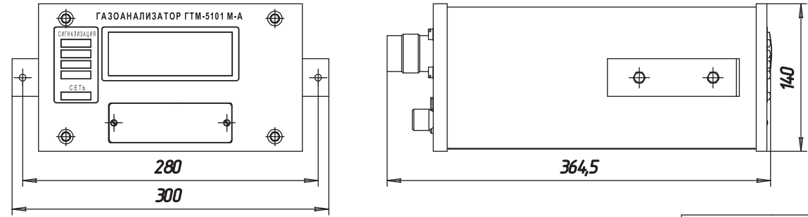
Разметка щита для установки газоанализатора
