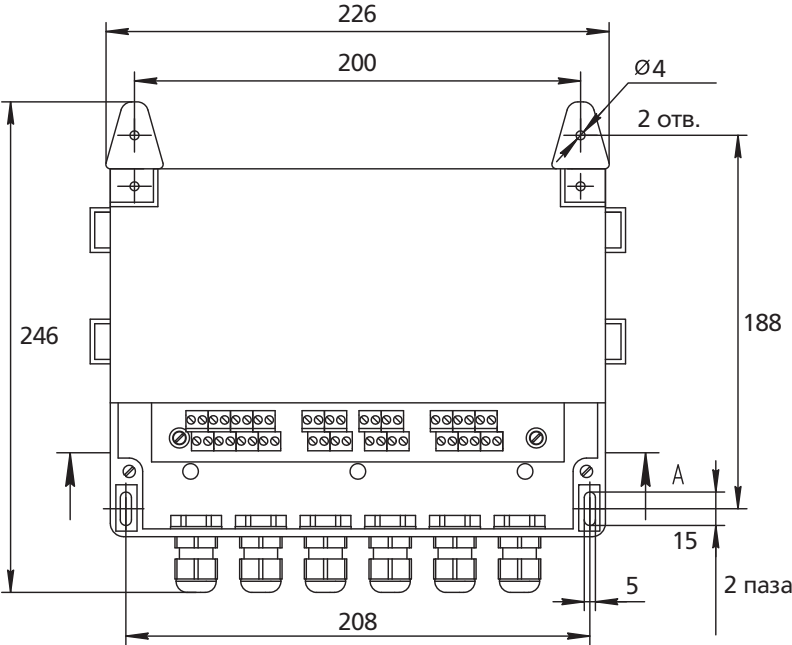
Диспетчерский пульт ДИСП Монтажный чертеж
