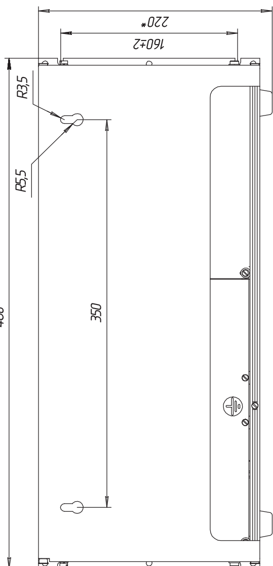
Внешний вид.
