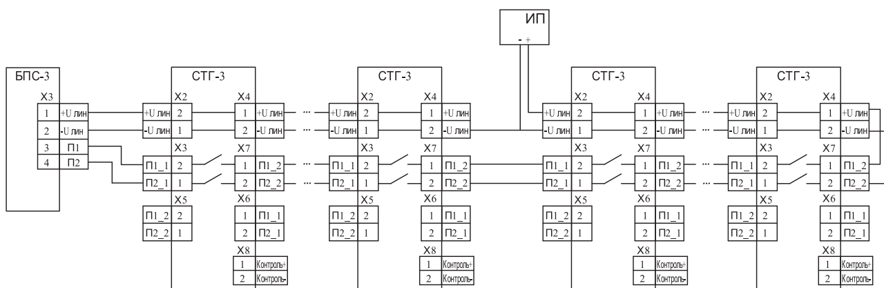
Схема шлейфового подключения сигнализаторов СТГ-3 к блоку БПС-3 и дополнительного источника питания
