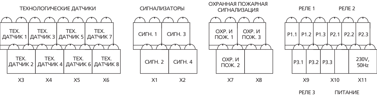
Подключение внешних устройств к выходам пульта
