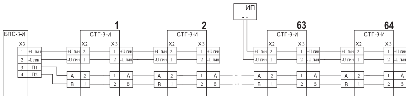
Схема шлейфового подключения сигнализаторов СТГ-3 к блоку БПС-3-И дополнительного источника питания
