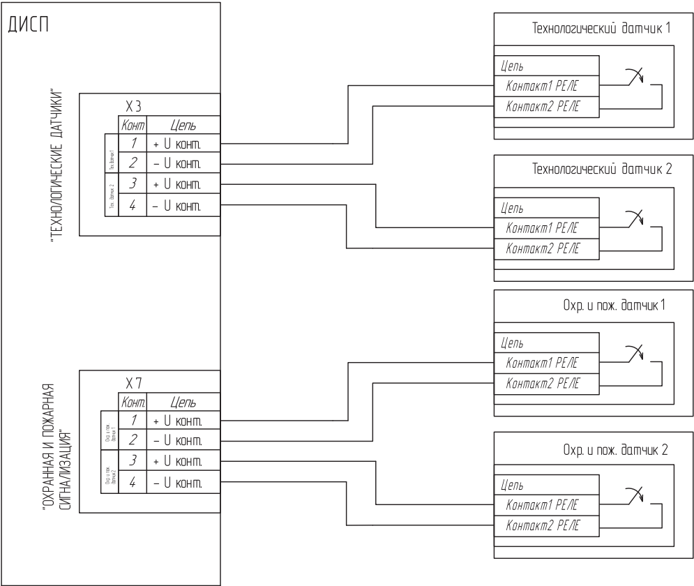
Схема подключения датчиков, приборов охранной и пожарной сигнализации к пульту
