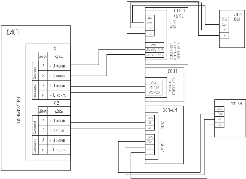
Схема подключения сигнализаторов горючих и токсичных газов к пульту
