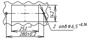
Разметка щита для установки газоанализатора
