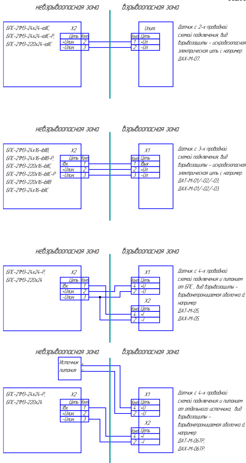
Рисунок 2.1 – Варианты подключения датчиков с различными схемами питания к блокам БПС-21МЗ-24х24-Р, БПС-21МЗ-24х16-ibПВ, БПС-21МЗ-24х16-ibПВ-Р, БПС-21МЗ-220х16-ibПС, БПС-21МЗ-24х16-ibПС-Р, БПС-21МЗ-220х24, БПС-21МЗ-220х16-ibПВ, БПС-21МЗ-24х16-ibПС, БПС-21МЗ-24х24-iaПС, БПС-21МЗ-24х24-iaПС-Р, БПС-21МЗ-220х24-iaПС
