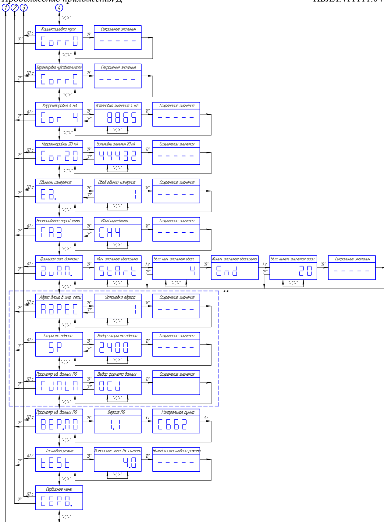
Продолжение рисунка Д.1 – Алгоритм режимов работы блоков БПС-21М3-24х24-Р, БПС-21М3-24х16-ibПВ-Р, БПС-21М3-24х16-ibПС-Р, БПС-21М3-220х24, БПС-21М3-220х16-ibПВ, БПС-21М3-220х16-ibПС, БПС-21М3-24х24-iaПС-Р, БПС-21М3-220х24-iaПС
