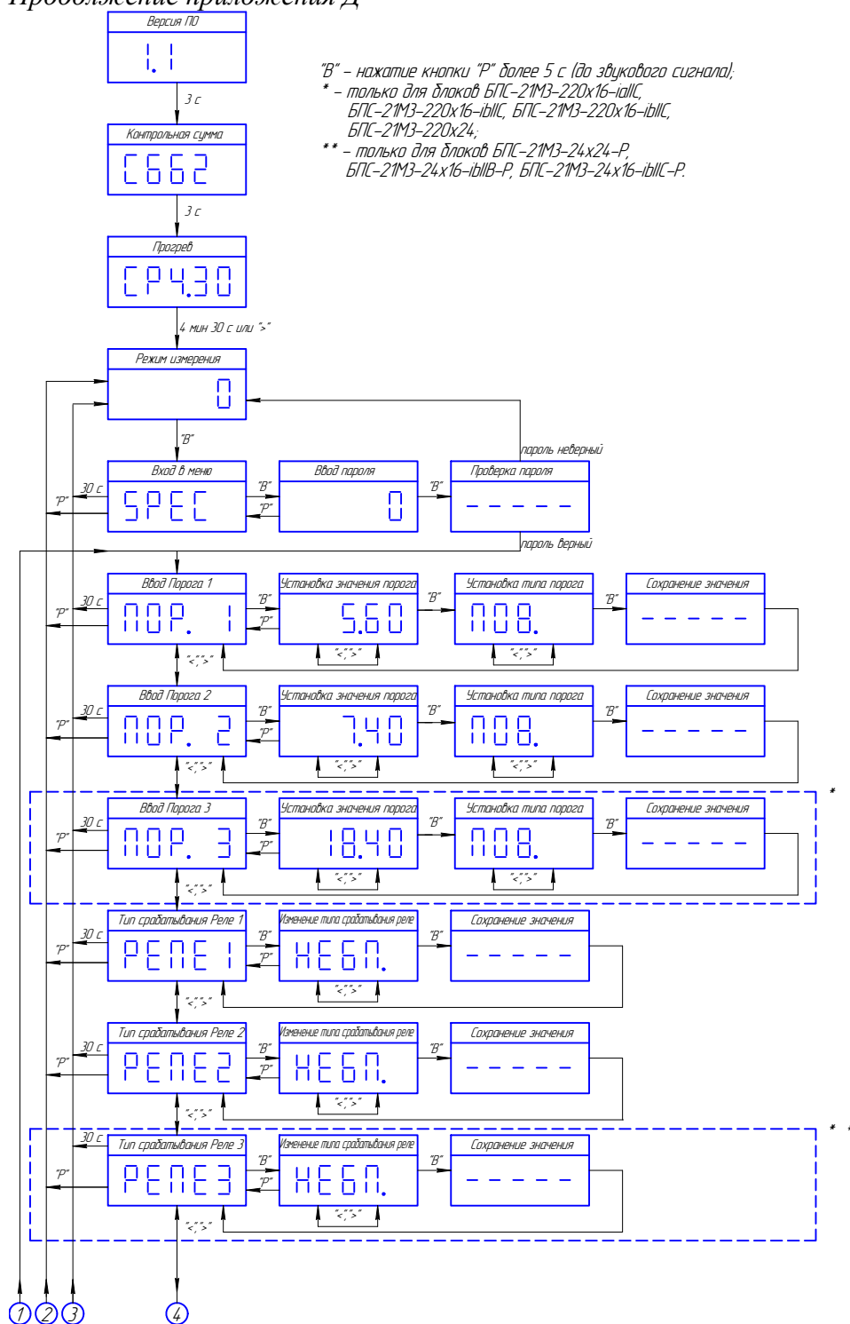
Рисунок Д.1 – Алгоритм режимов работы блоков БПС-21М3-24х24-Р, БПС-21М3-24х16-ibПВ-Р, БПС-21М3-24х16-ibПС-Р, БПС-21М3-220х24, БПС-21М3-220х16-ibПВ, БПС-21М3-220х16-ibПС, БПС-21М3-24х24-iaПС-Р, БПС-21М3-220х24-iaПС
