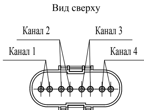
Рисунок 3.2 – Последовательность расположения каналов в маске для ПГС ИБЯЛ.304131.056
