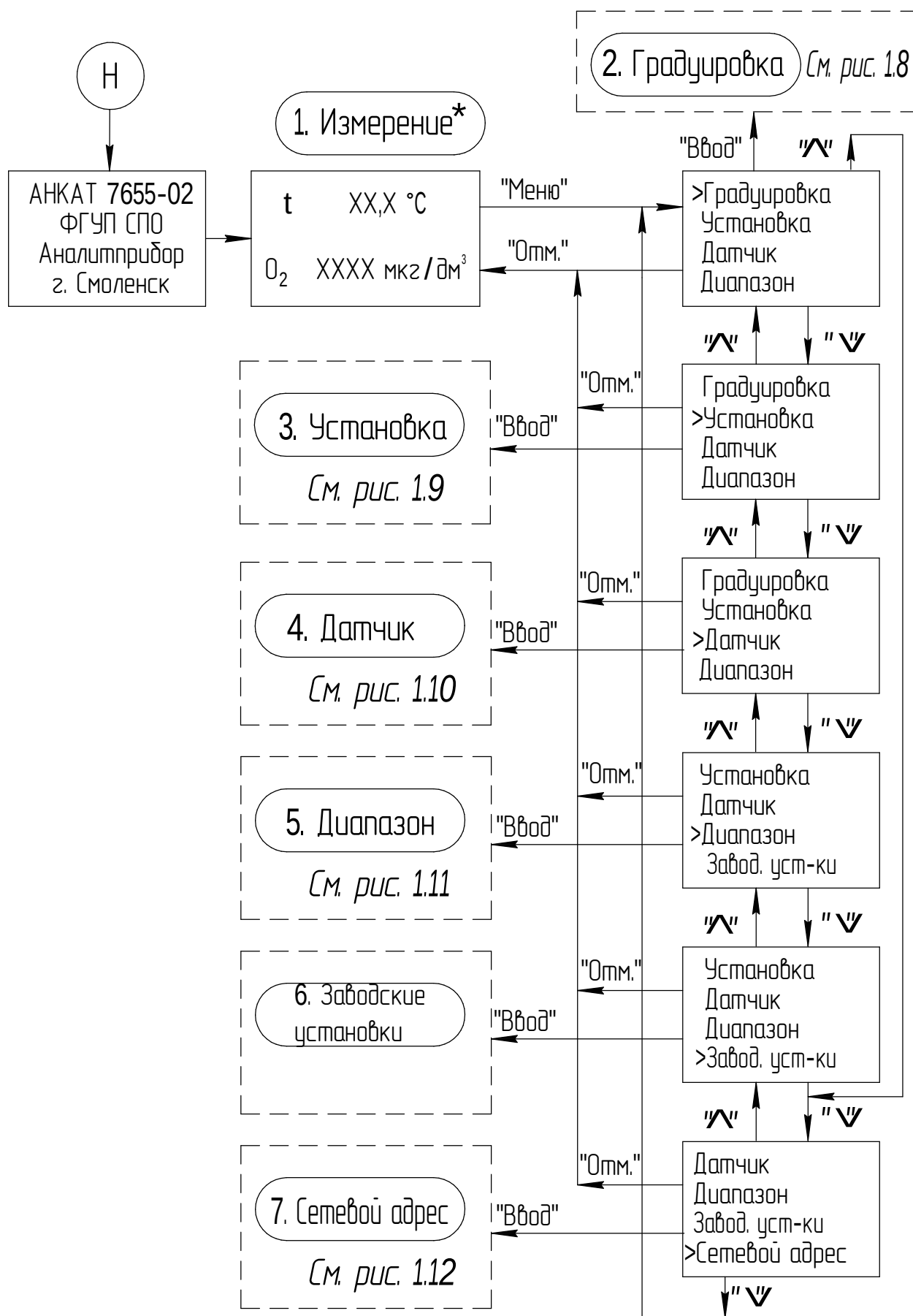
Рисунок 1.7 - Основное меню режимов работы АНКАТ 7655-02
