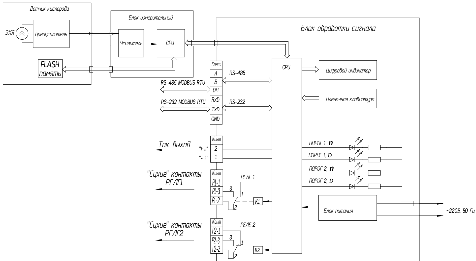
Рисунок 1.5 - Анализатор АНКAT 7655-02. Схема функциональная
