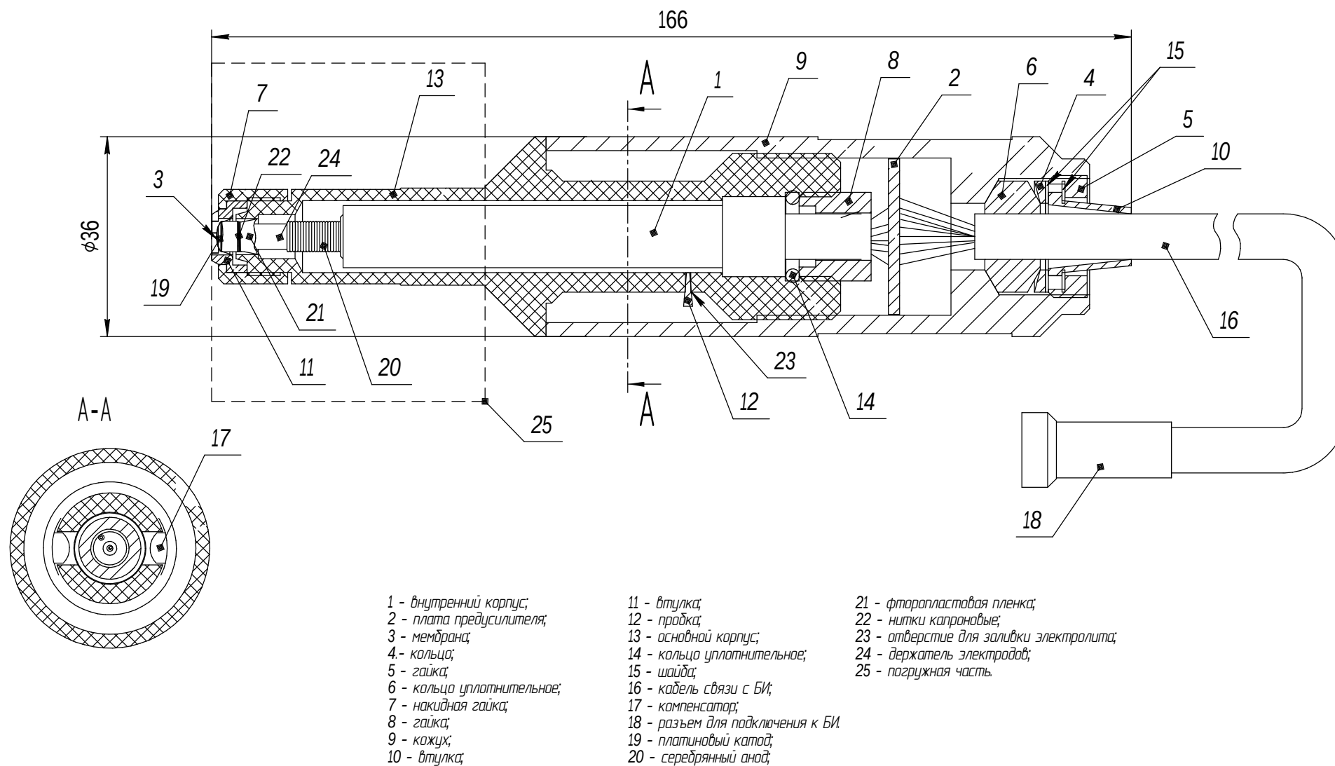
Рисунок 1.3 - Внешний вид и конструкция датчика
