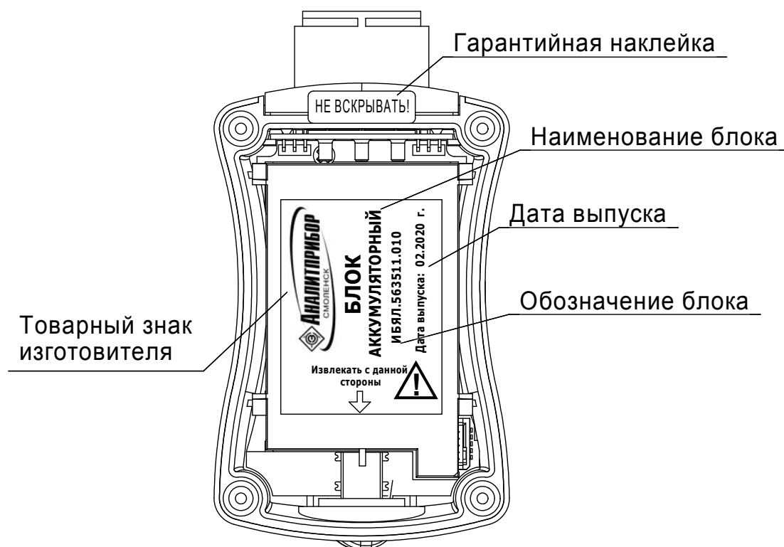
Рисунок 1.6 – Маркировка аккумуляторного блока и расположение гарантийной (пломбировочной) наклейки
