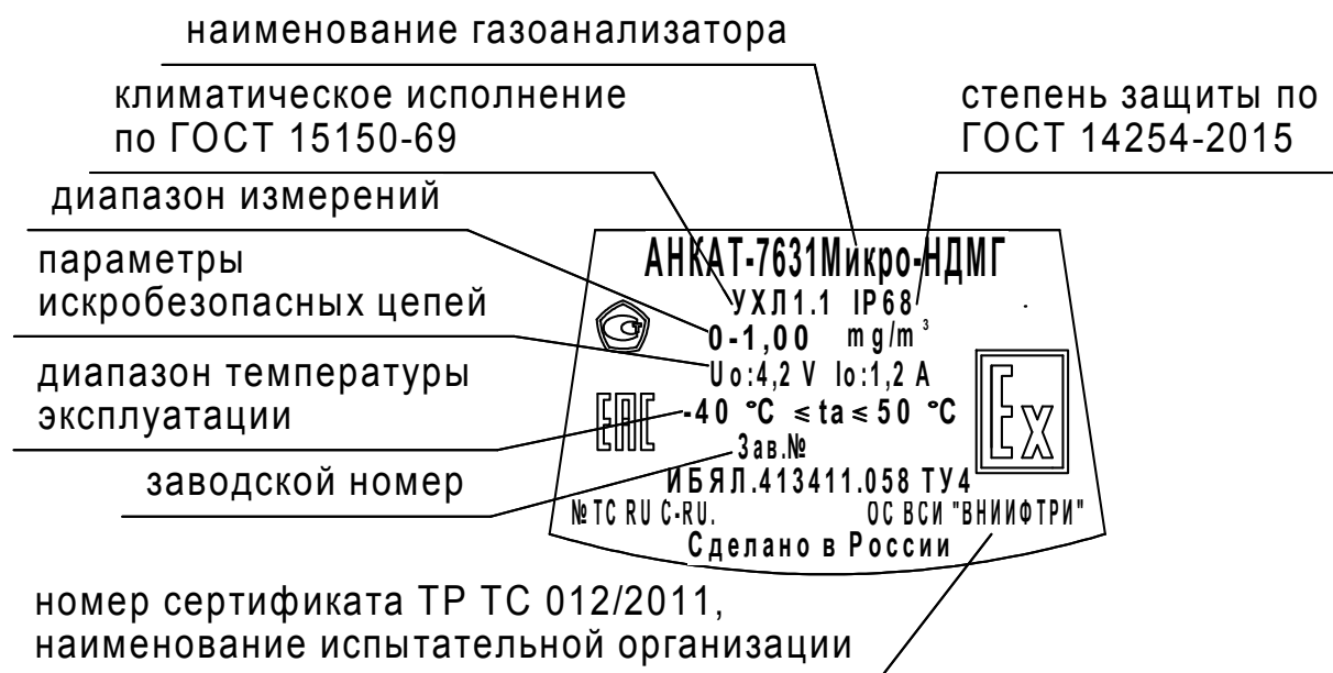
Рисунок 1.5 – Маркировочная табличка
