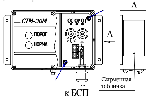
Рисунок Г.4 – БД сигнализаторов СТМ-30М-50ДБ, -51ДБВ, -53ПБВ
