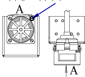
Рисунок Г.3 – БД сигнализаторов СТМ-30М-00ДЦ, -02ДЦВ, -04ПЦВ, -07ДЦВ
