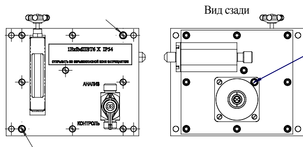
Рисунок Г.2 - ВД сигнализаторов СТМ-30М-04ПЦВ, -53ПБВ с принудительным отбором пробы
