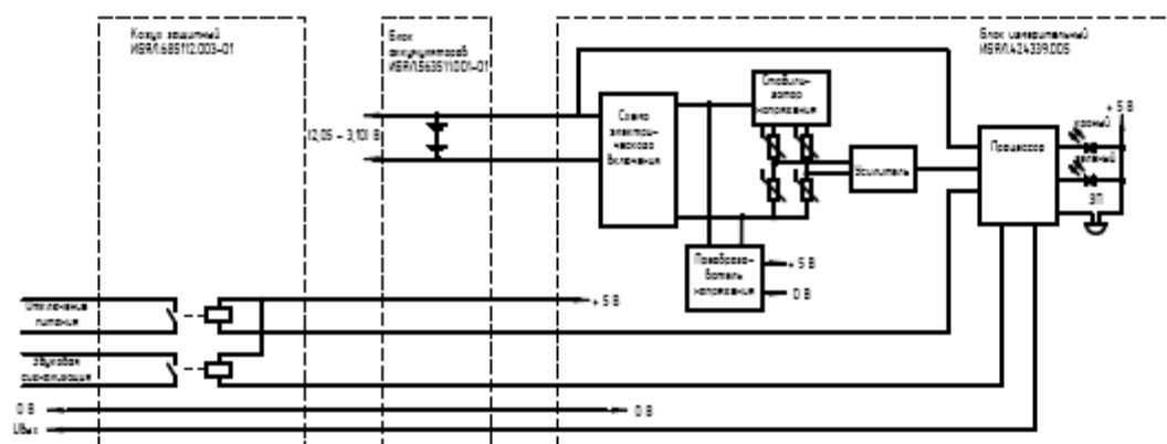
Рисунок 11 – Сигнализаторы СТШ. Схемы электрические функциональные
