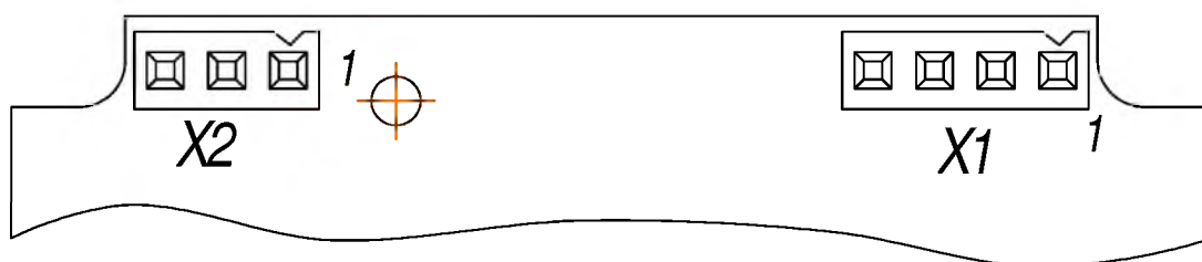
Рисунок В.2 – Расположение разъема X1 на плате модуля измерений и индикации ИБЯЛ.468157.007
