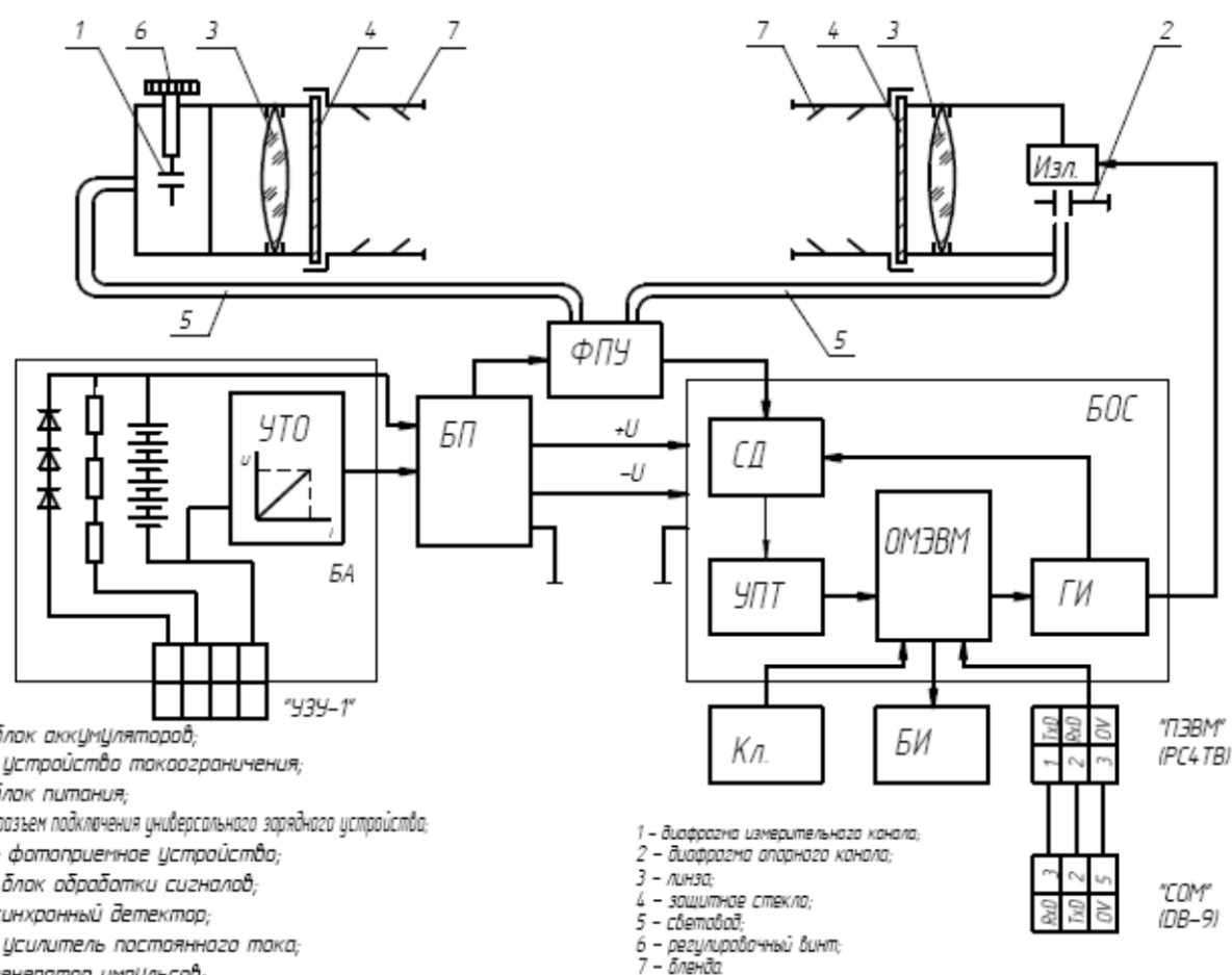
Рисунки 4.2 – Измеритель ИКВ4-В3. Схема функциональная
