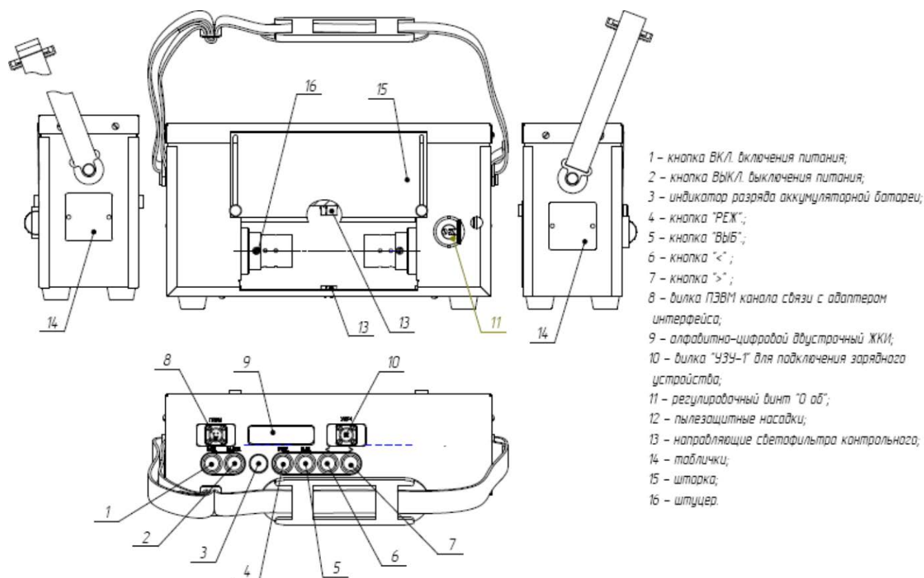
Рисунок 4.1 – Измеритель ИКВ4-В3. Внешний вид
