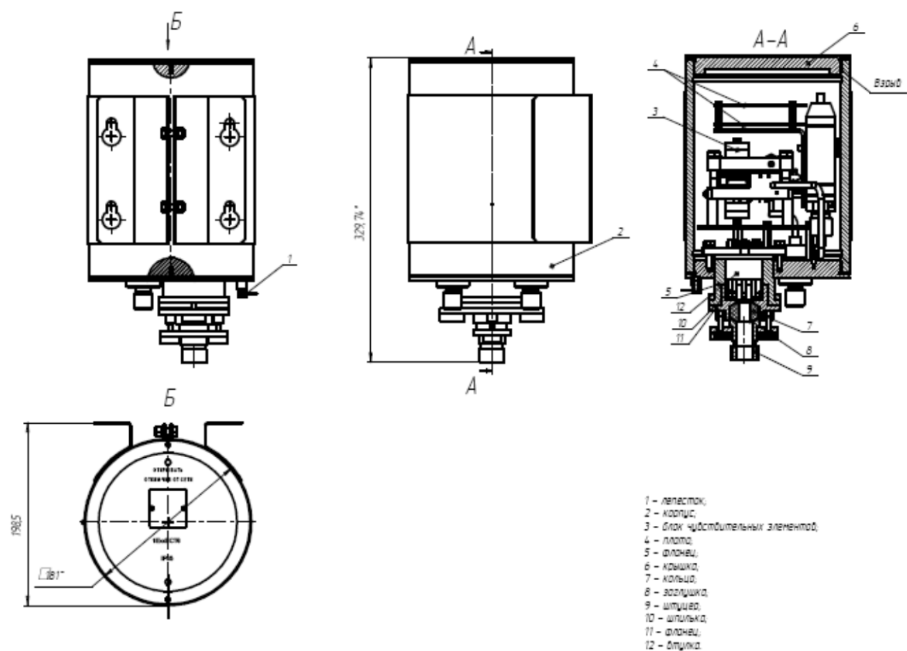
Рисунки 1.2 – Преобразователь лавинный. Внешний вид
