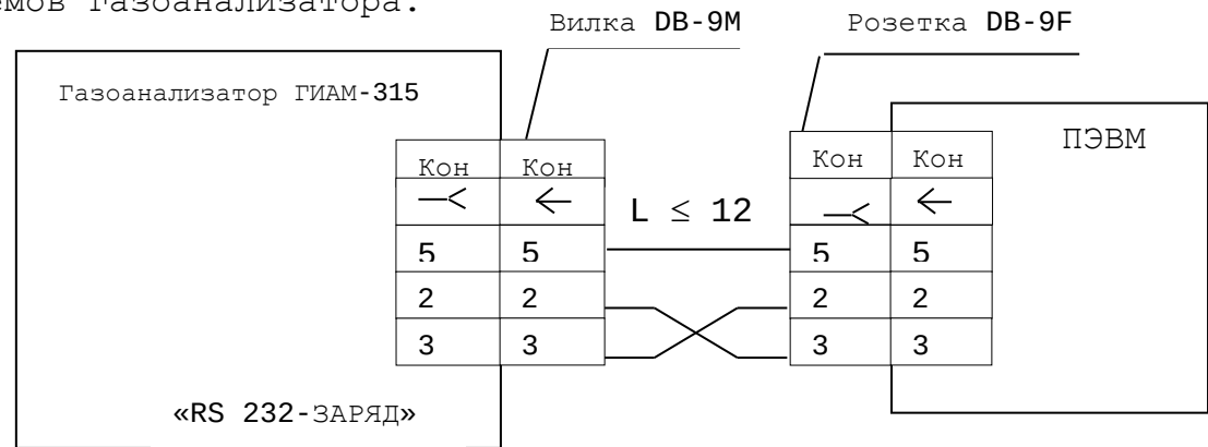
Рисунок 2.1 – Схема подключения газоанализатора ГИАМ-315 к ПЭВМ
