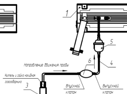
б) принудительный забор пробы с помощью газозаборника ИБЯ/Л418311.043 (температура окружающего воздуха от минус 10 до 40 °С)
