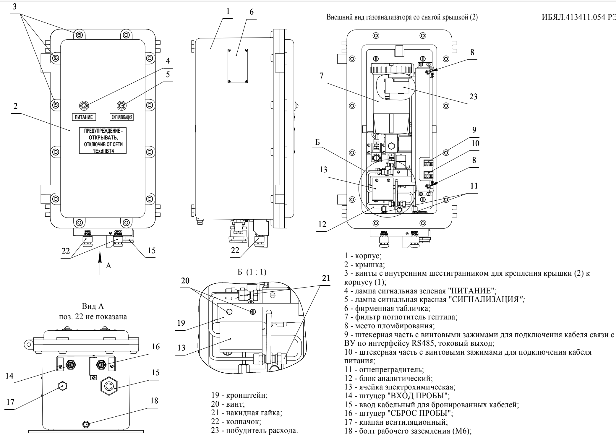
Рисунок 1.1 - Датчик-газоанализатор паров КРТ ДАРТ. Внешний вид
