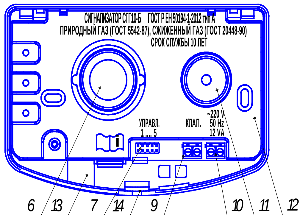
Рисунок 11 (б) - Сигнализаторы горючих газов СТ10-Б Внешний вид
