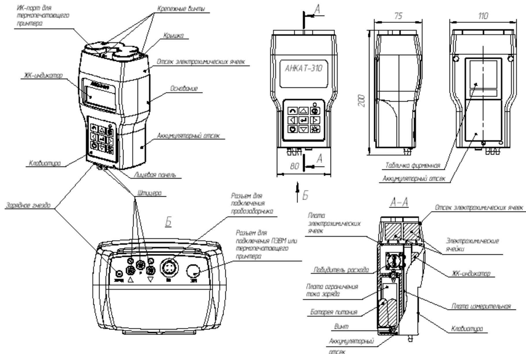
Рисунок 1.1 – Газоанализаторы АНК-310. Внешний вид
