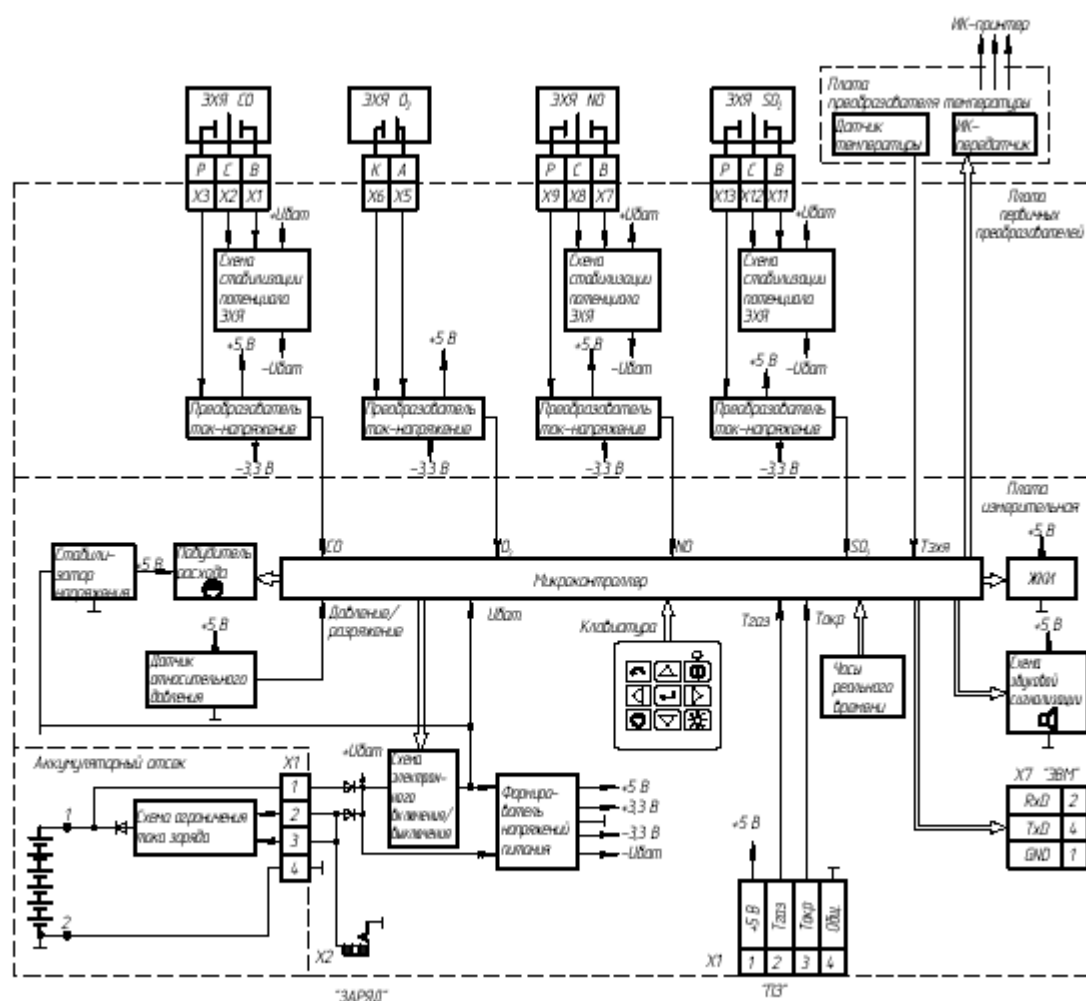
Рисунок 12 – Газоанализаторы АНКАТ-310. Функциональная схема
